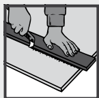
Figure 1 : Rainurer la plaque pour la casser facilement
