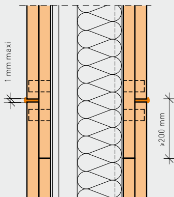
1 re couche/couche intérieure fixée sans colle 2 e couche/couche extérieure collée
