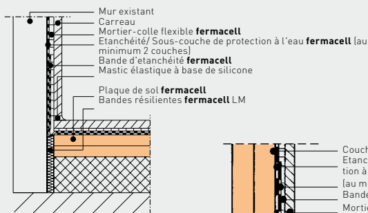
Raccord d'angle exposé aux projections
